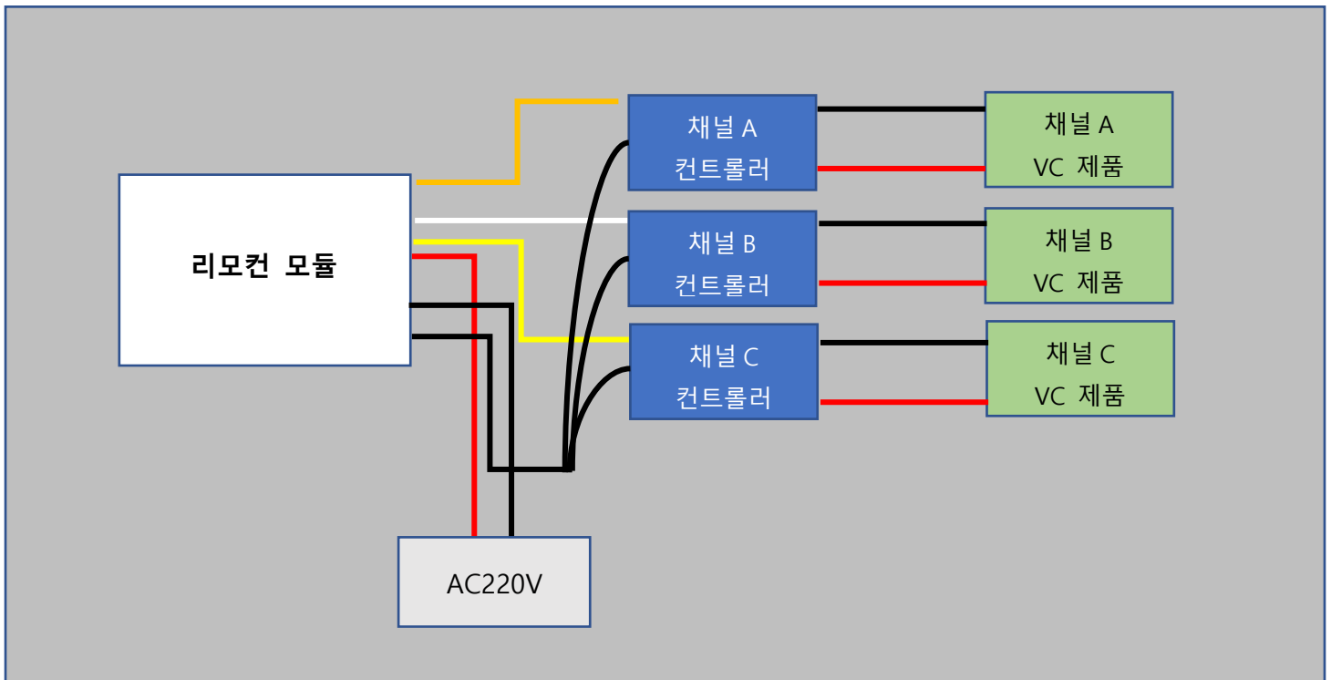
[리모컨 모듈 배선 연결]
